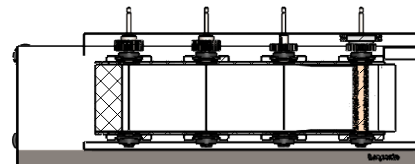
SECTION D-D
