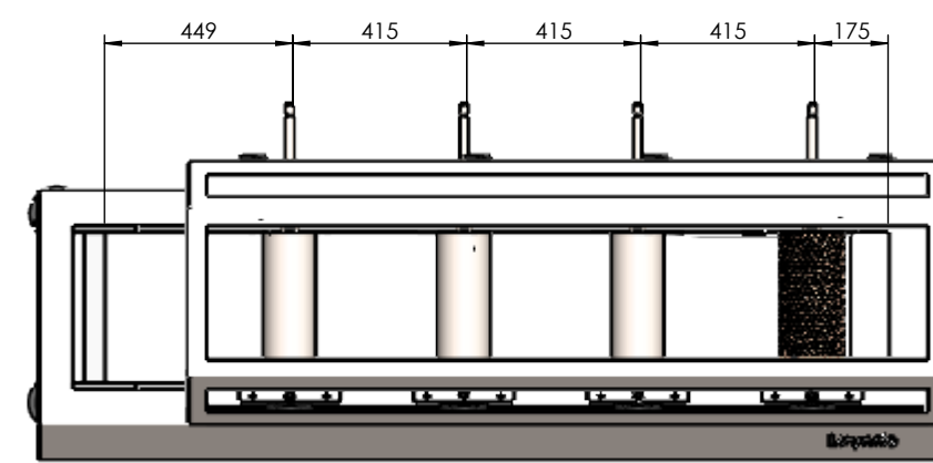
SECTION A-A
